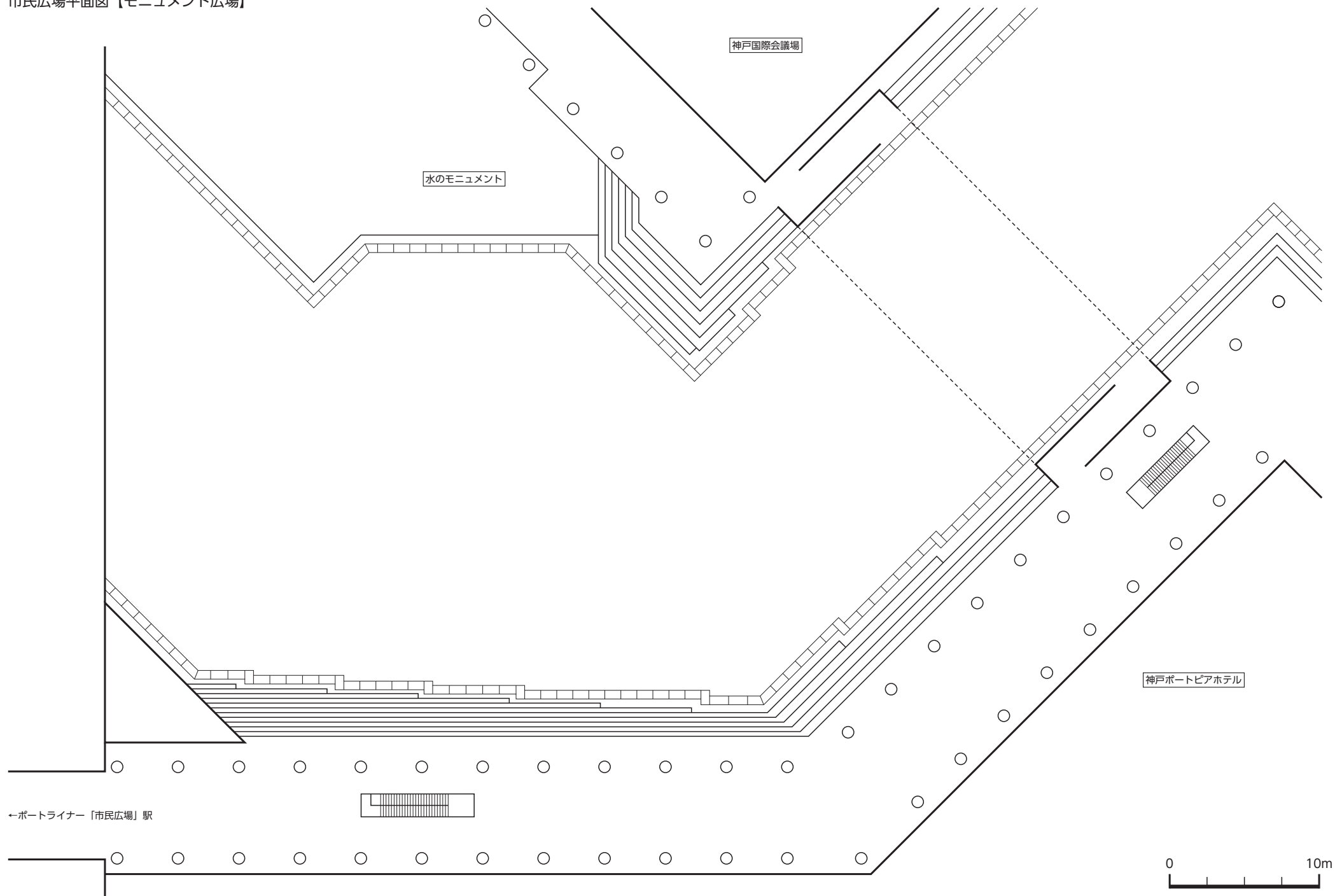
市民広場平面図【モニュメント広場】
