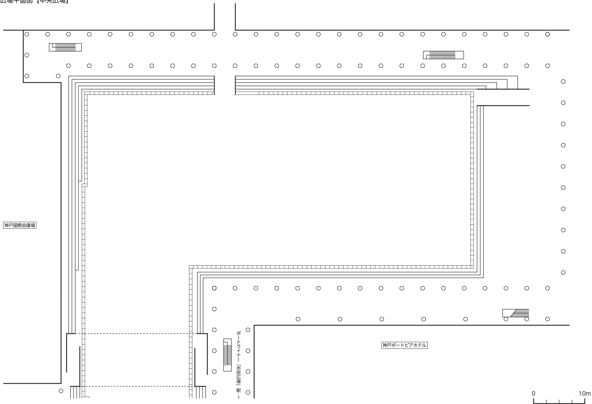
市民広場平面図【中央広場】
