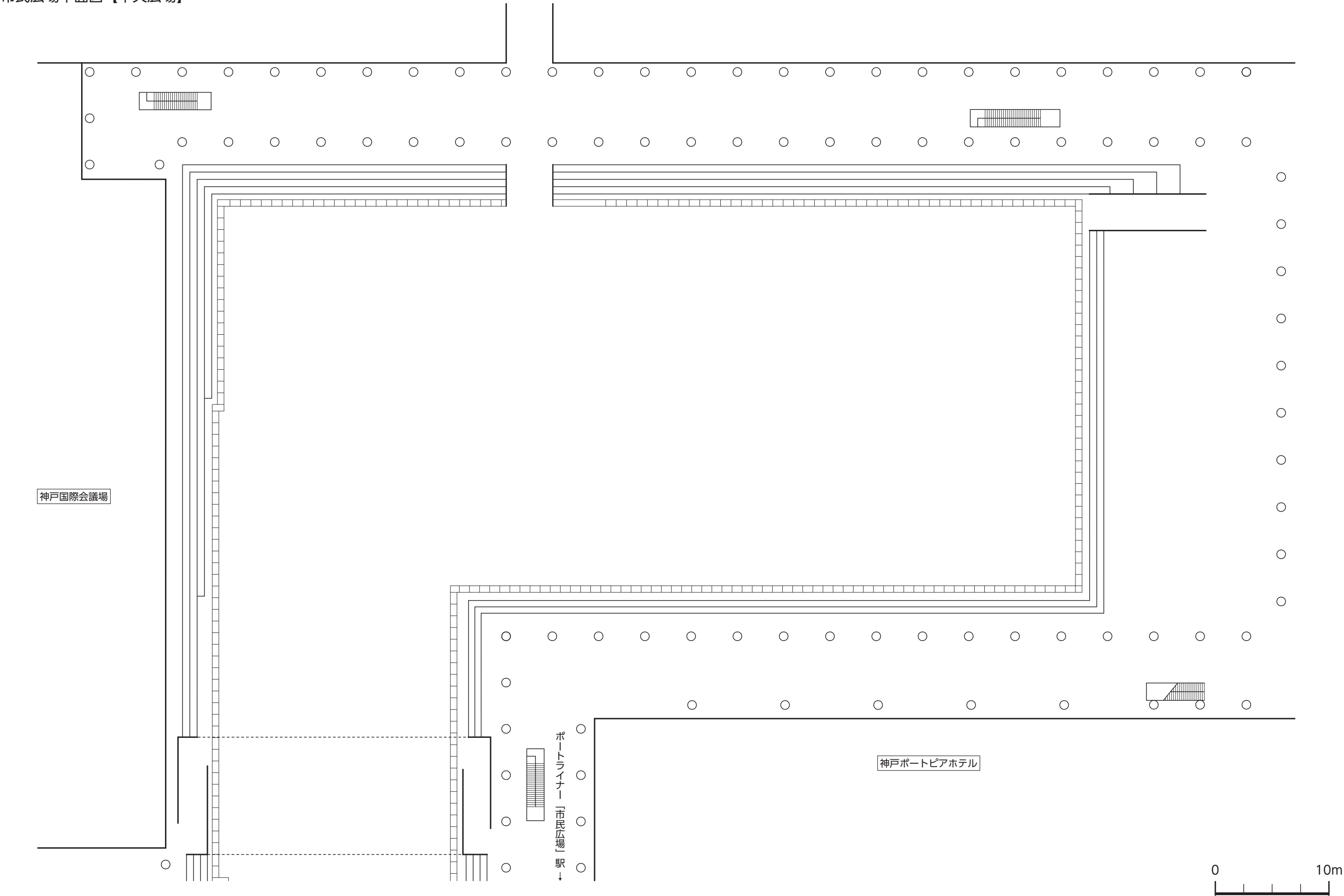
市民広場平面図【中央広場】
